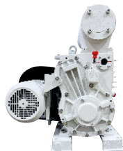
АВПл-20Д НАСОС ВАКУУМНЫЙ ПЛУНЖЕРНЫЙ (версия маслоотделителя без фильтра)
